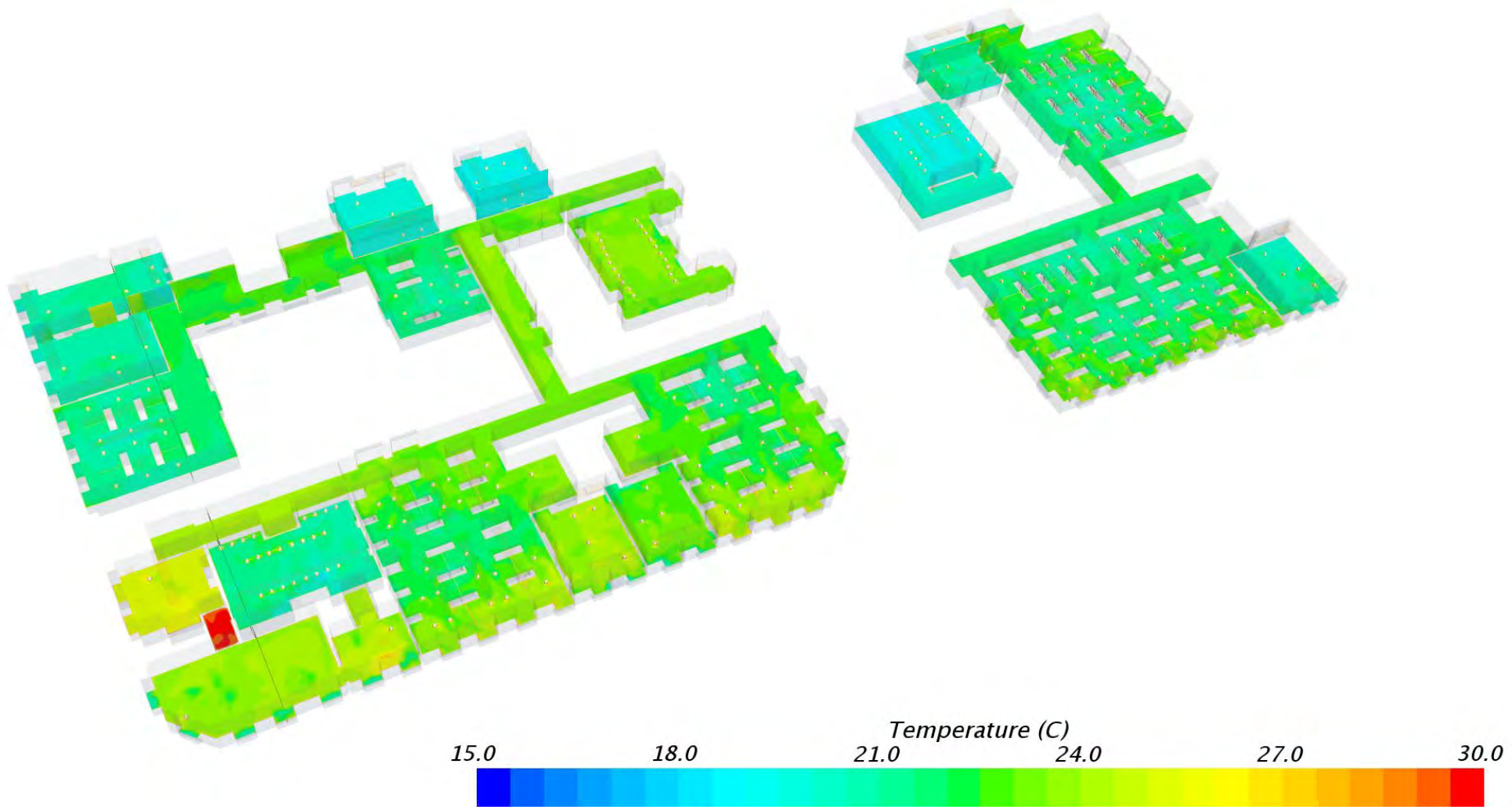
Распределение температуры воздуха на уровне 1,6 метра от пола
