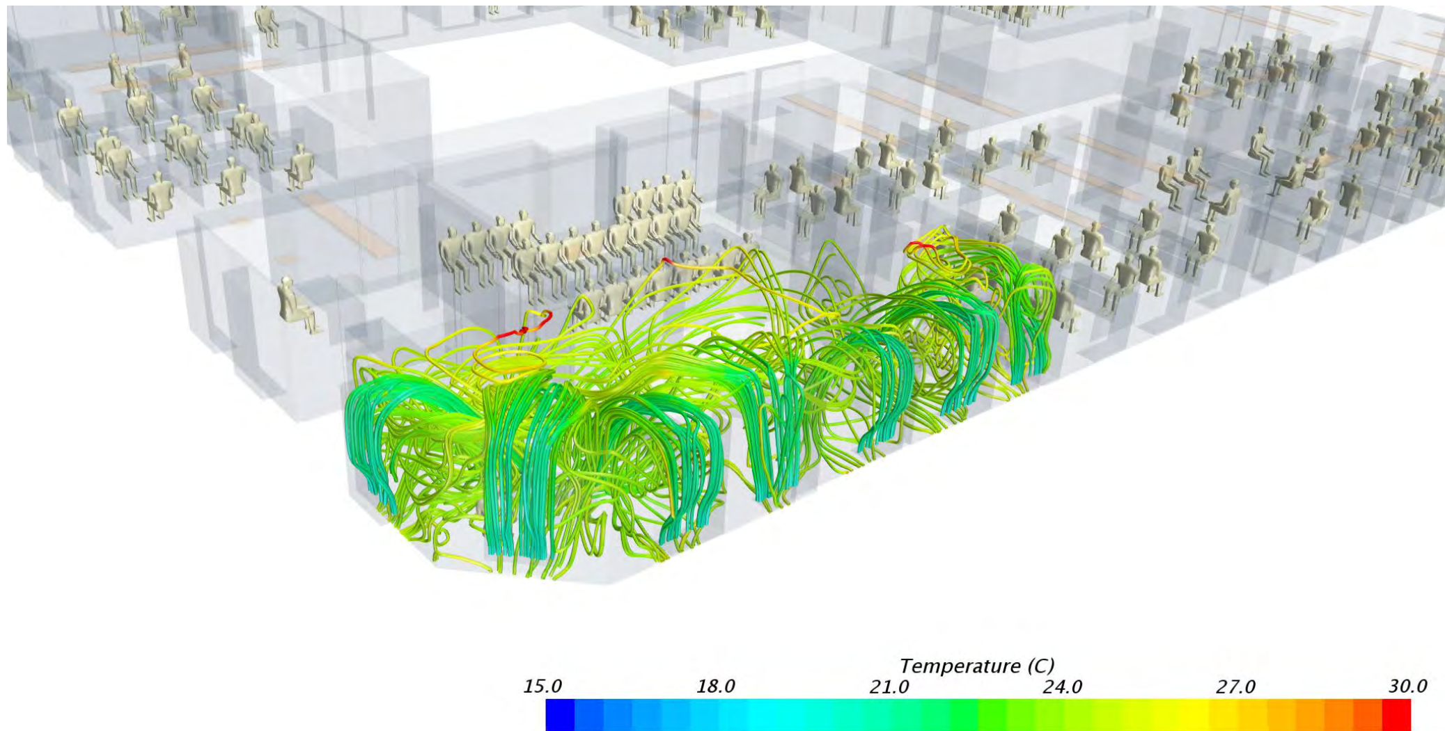
Линии тока воздуха от климатических балок.
